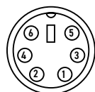
Mini DIN 6-pol.
