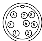
Mini DIN 8-pol.
