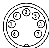
DIN 7-pol.
