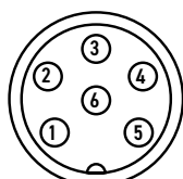
DIN 6-pol.
